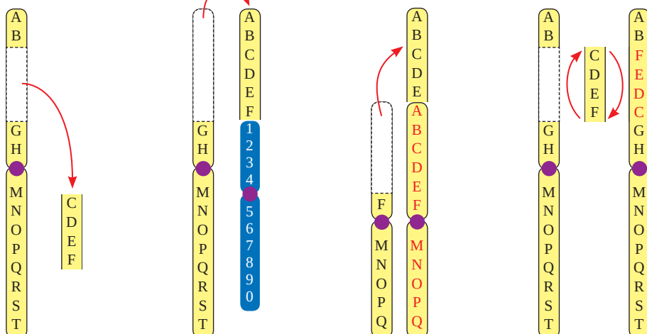
شکل ۴- انواع ناهنجاری های ساختاری در فام تن ها
