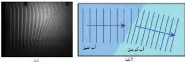
(الف) طرحی از شکست امواج سطحی در مرز آب عمیق و آب کم عمق در (ب) تست موج و آب تصویری واقعی از شکست امواج سطحی در تست موج
