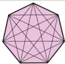
Heptagon ۷ ضلعی
