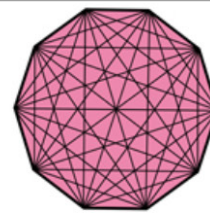
Decagon ۱۰ ضلعی
