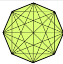
Octagon ۸ ضلعی
